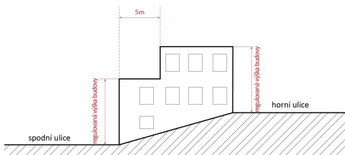
Obr. 2. Obr. 1. Regulovaná výška budovy pokud se budova nachází v situaci, kdy se dotýká na protilehlých stranách dvou komunikací, jež jsou na jiných výškových úrovních.
