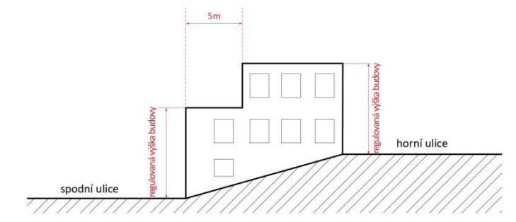
Obr 2. Regulovaná výška budovy pokud se budova nachází v situaci, kdy se dotýká na protilehlých stranách dvou komunikací, jež jsou na jiných výškových úrovních.
