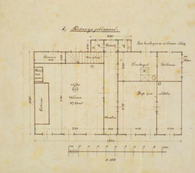
Půdorys školy po rekonstrukci v roce 1870 (školní kronika, díl 1, s. 22).
